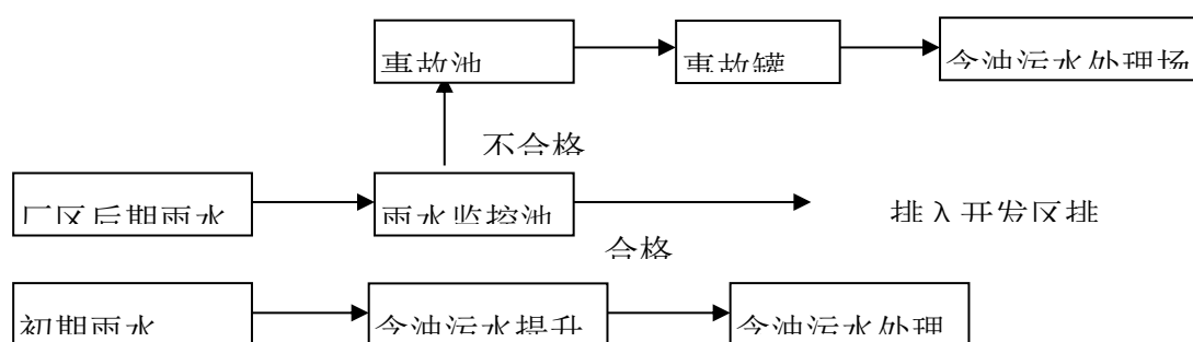
图 4-11 全厂雨排系统示意图
